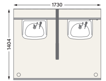
MU-MM 手洗+手洗 W1730×D1404×H1950 / 約 130kg
