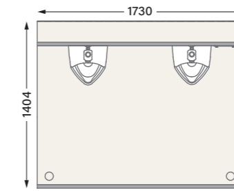
MU-SS 小便+小便 W1730×D1404×H1651 / 約 130kg
