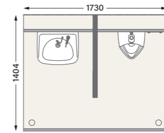
MU-MS 手洗+小便 W1730×D1404×H1950 / 約 140kg
