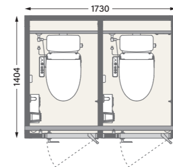
MU-WW 洋式+洋式 W1730×D1404×H2090 / 約 300kg
