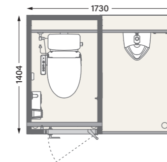
MU-WS 洋式+小便 W1730×D1404×H2090 / 約 230kg
