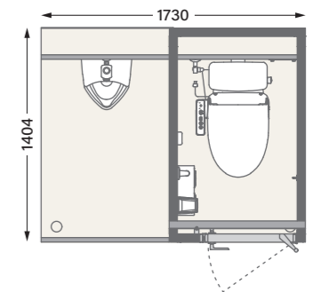
MU-SW 小便+洋式 W1730×D1404×H2090 / 約 230kg
