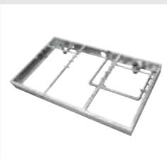
排水ユニット ※お客様にて現地取付となります。 ※水洗のみ対応となります。 2室タイプ:W1910×D1630×H250 3室タイプ:W2850×D1630×H250
