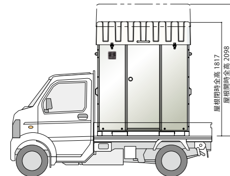
軽トラック積載時全高2500未満(道路交通法)
