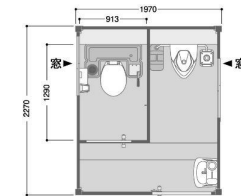
⑫ 便房内寸法900×900mm以上 (室内寸法913×1290mm)
