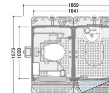
⑫ 便房内寸法900×900mm以上 (室内寸法1641×1008mm)
