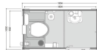
⑫ 便房内寸法900×900mm以上 (室内寸法1834×932mm)
