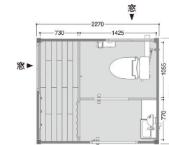
⑫ 便房内寸法900×900mm以上（室内寸法1505×1425mm）
