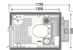
⑫ 便房内寸法900×900mm以上 (室内寸法1306×920mm)
