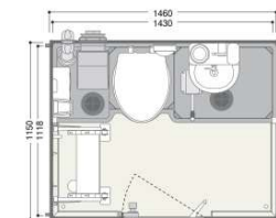
⑫ 便房内寸法900×900mm以上 (室内寸法1430×1118mm)
