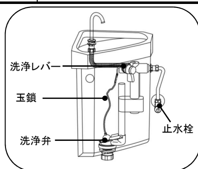
CTiX、CTWiX ロータンク
