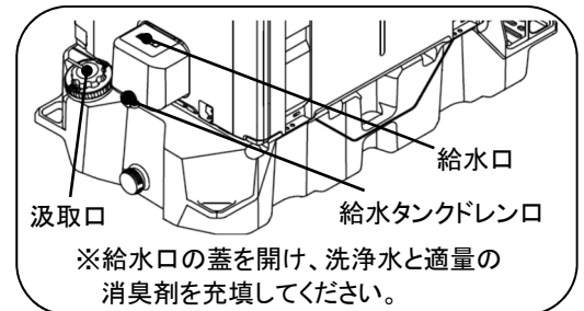
本体後部(CTiXF4)
