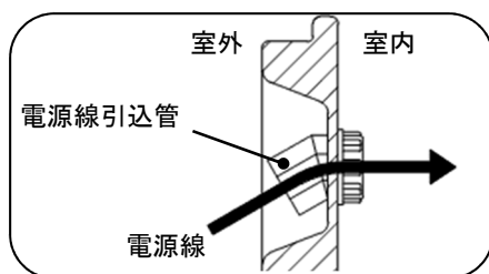
電源線引込口
