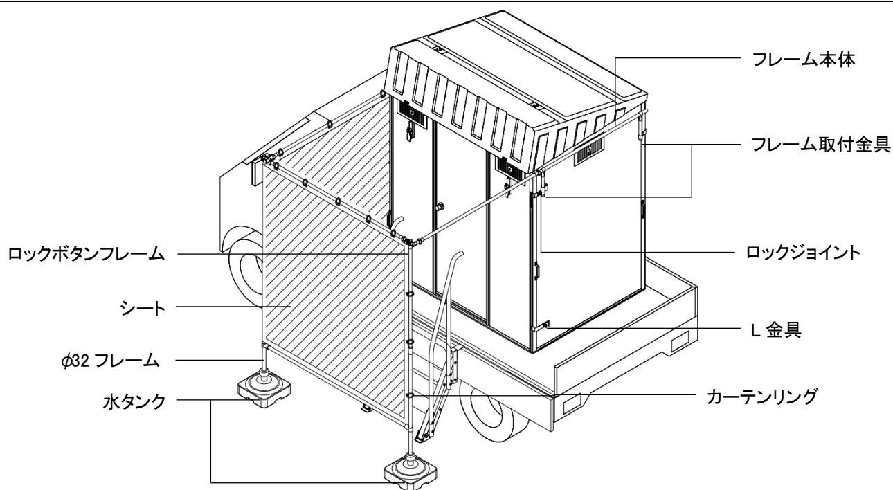
TU-LP(車載トイレパーテーション)
