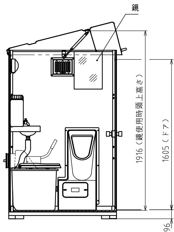
側面図 (内装)
