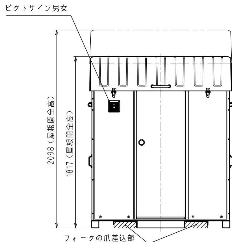
正面図
