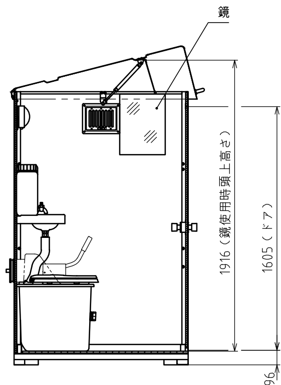
側面図 (内装)
