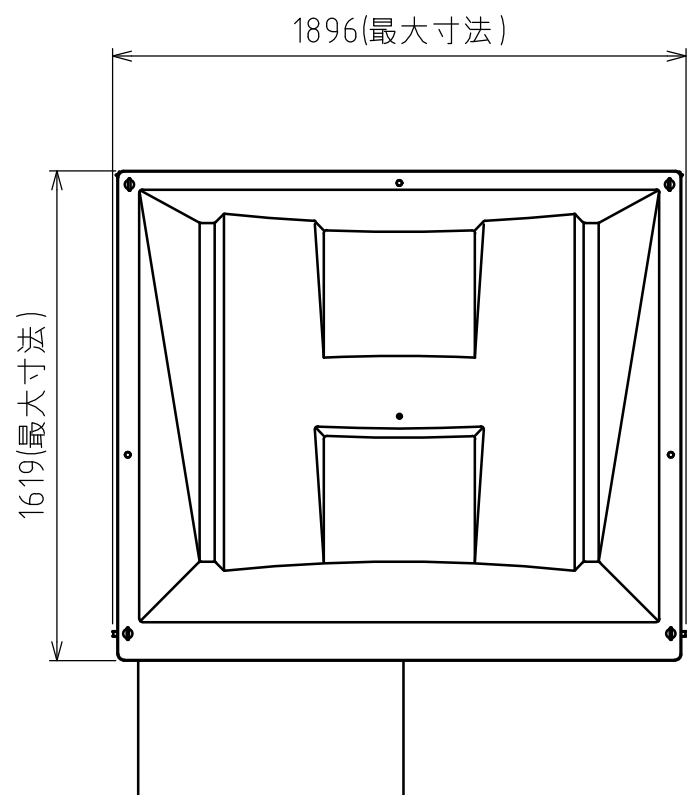
屋根伏図
