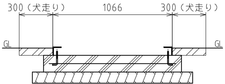
断面BB
