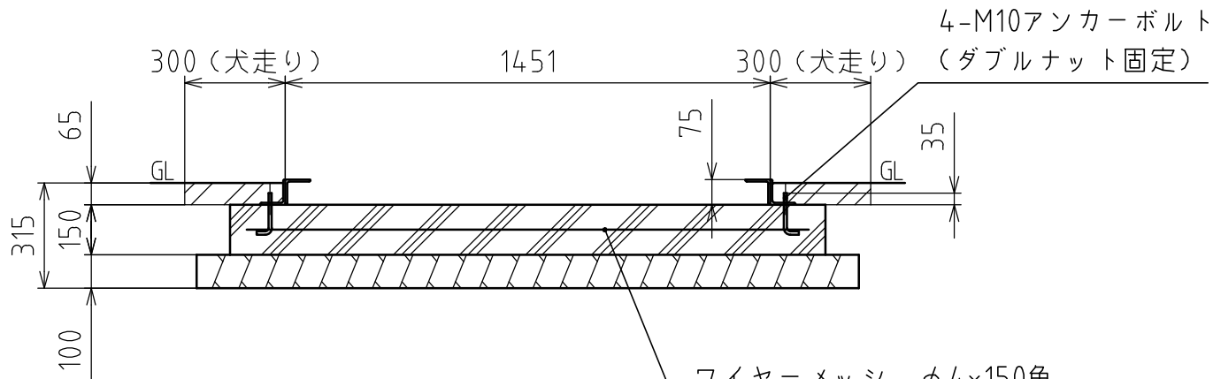
断面AA
