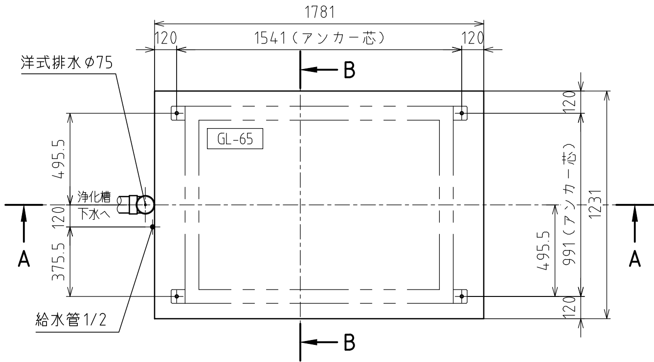
基礎平面図
