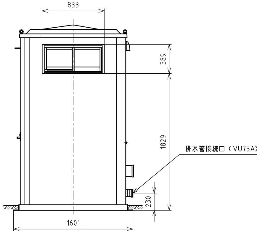
右側面図
