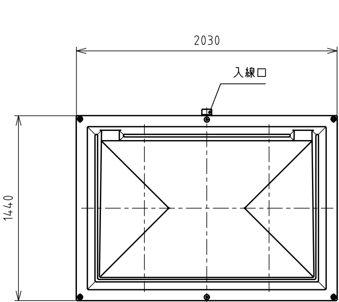
屋根伏図
