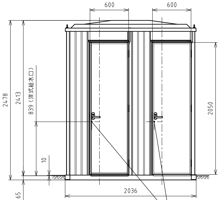
正面図
