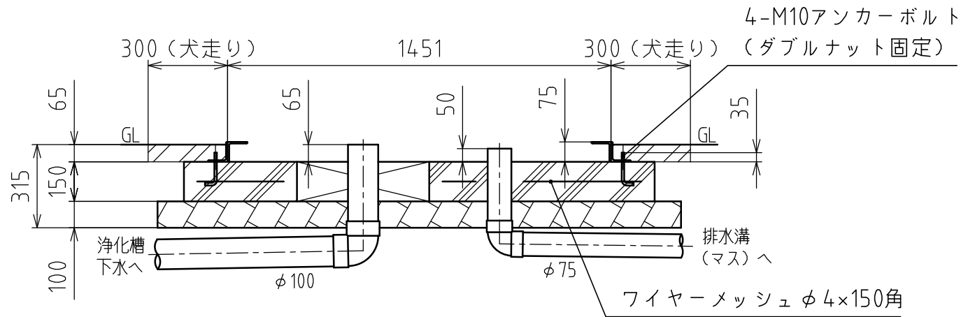
断面AA
