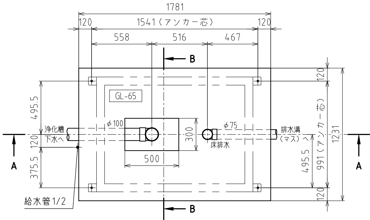
基礎平面図
