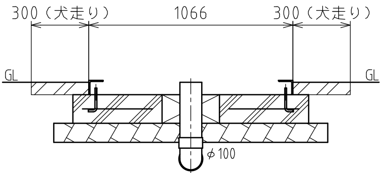
断面BB
