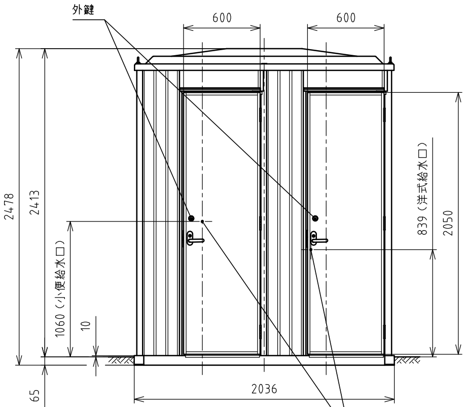
正面図
