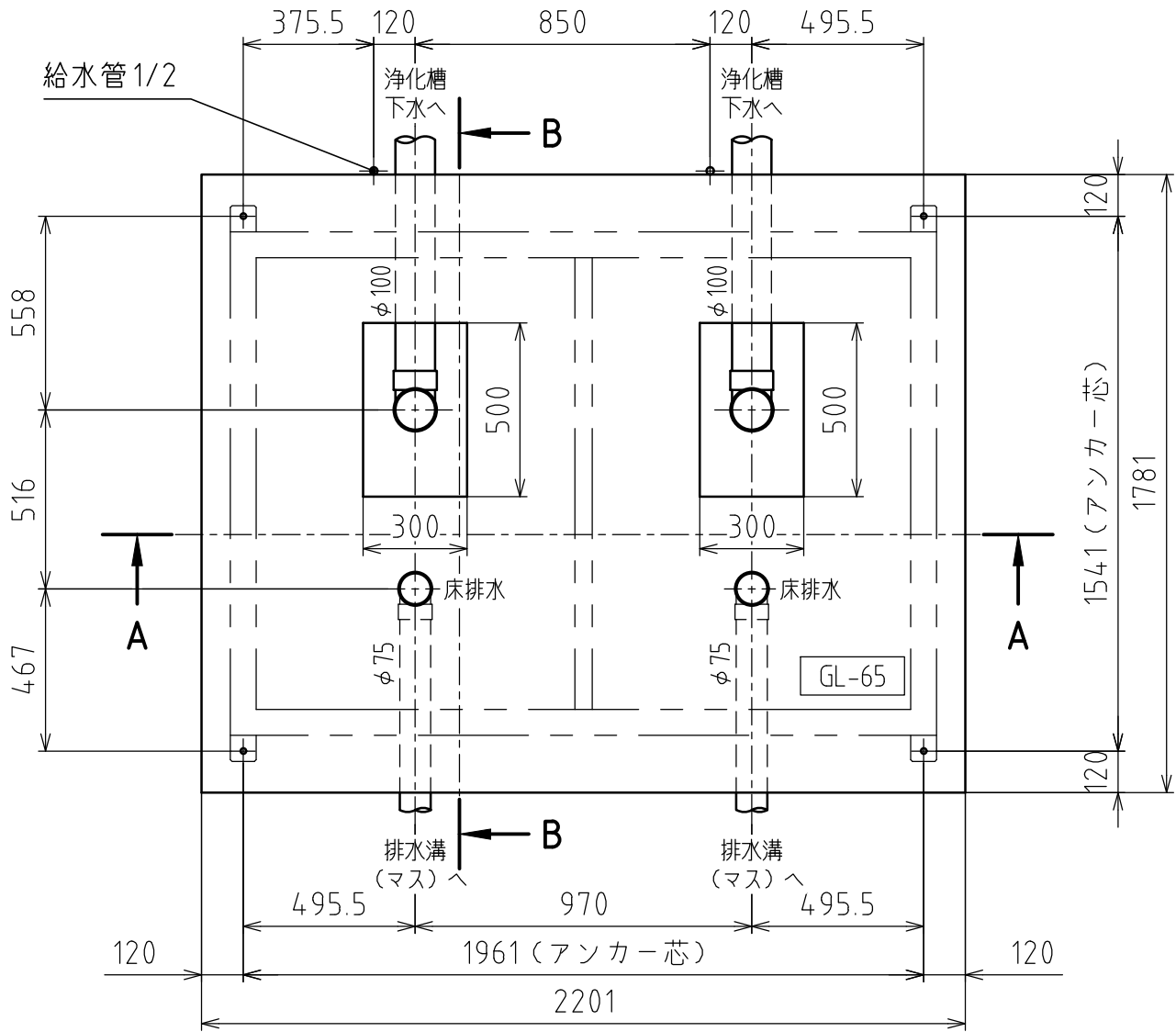
基礎平面図
