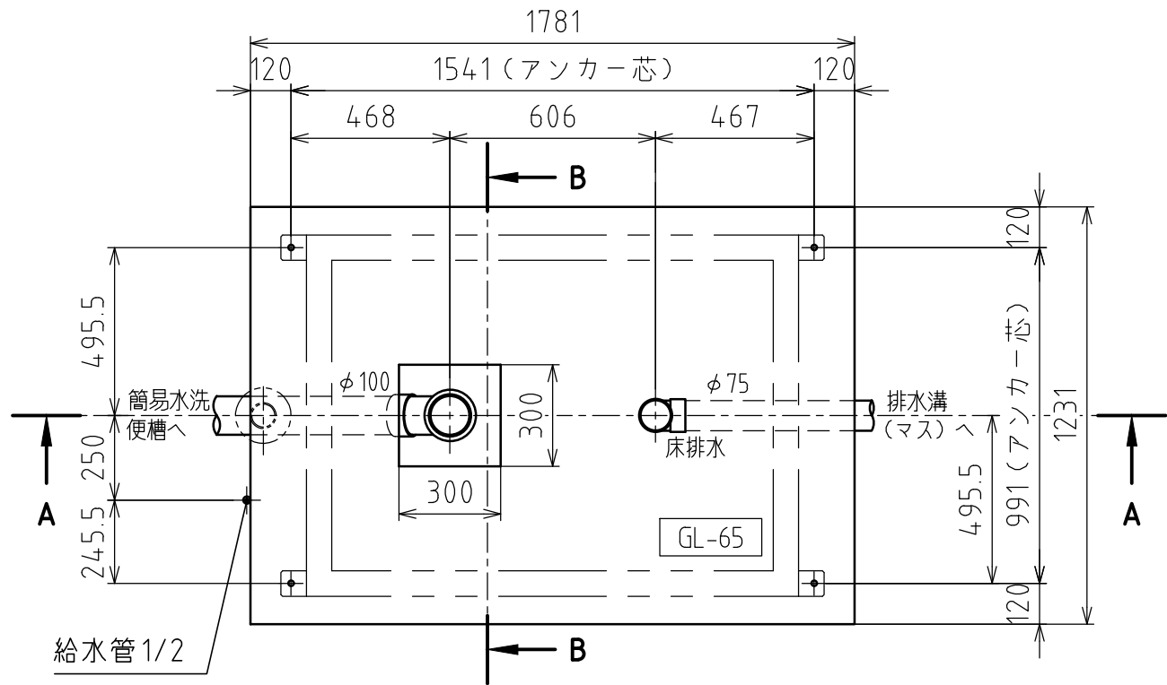
基礎平面図
