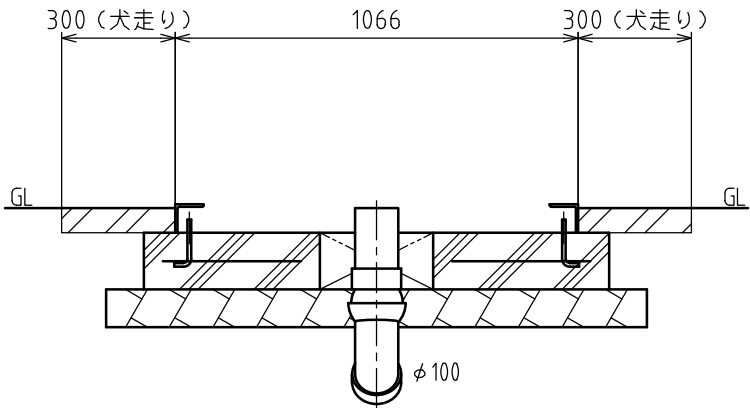
BB断面図
