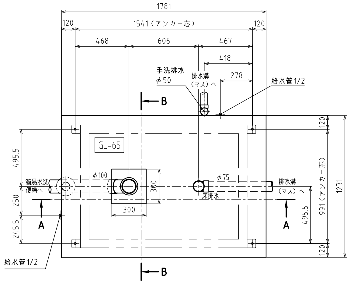
基礎平面図
