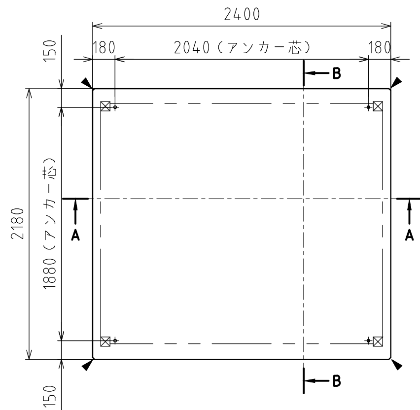
基礎平面図
