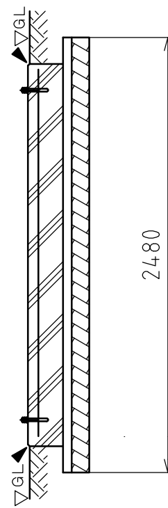
B-B断面図
