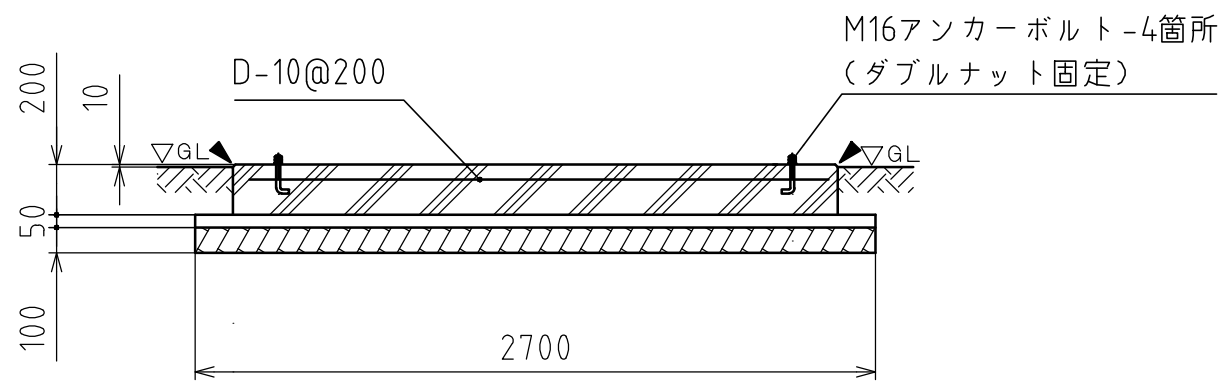
A-A断面図
