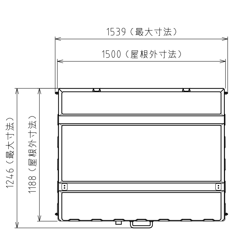
屋根伏図
