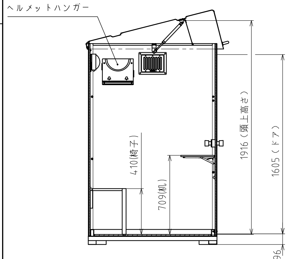
側面図 (内装)
