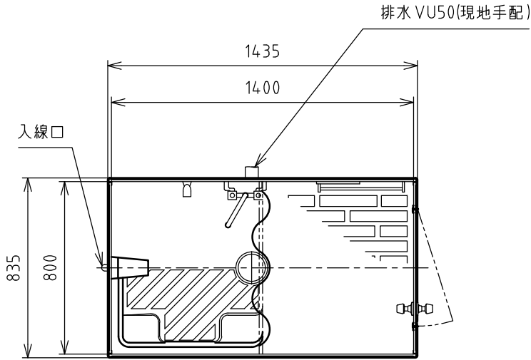
平面
