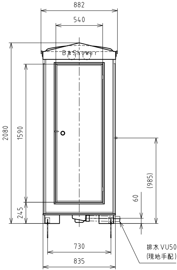
正面
