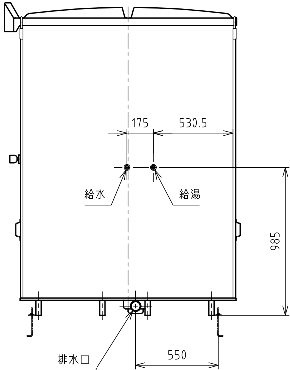
右側面
